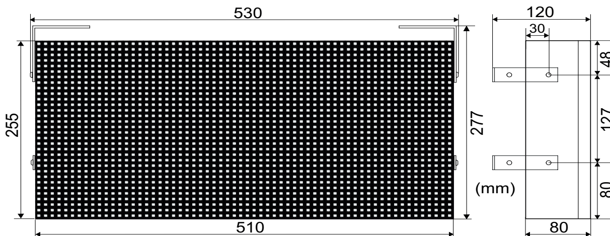
Fig. 3 DISCRSE dimensions
